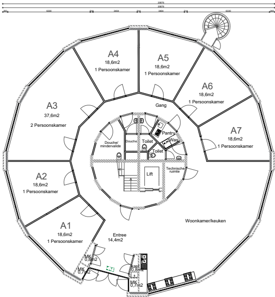
BEGANE GROND (PEIL)
