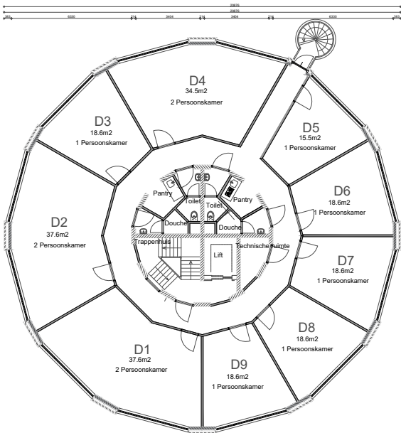
3e VERDIEPING (9600+P)
