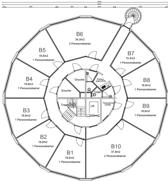
1e VERDIEPING (3200+P)
