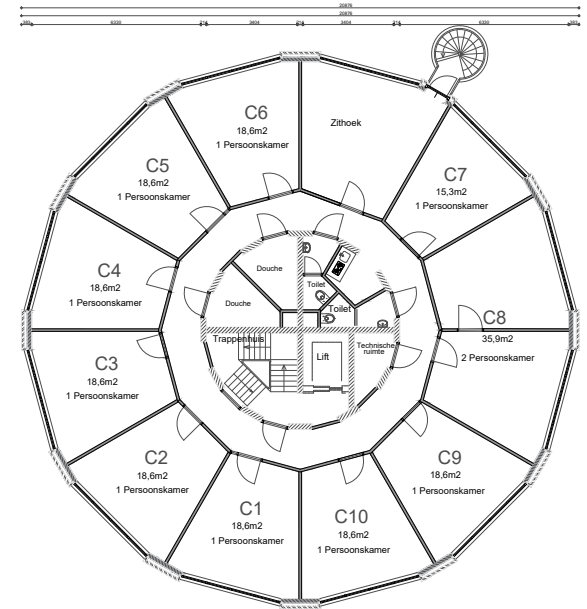
2e VERDIEPING (6400+P)
