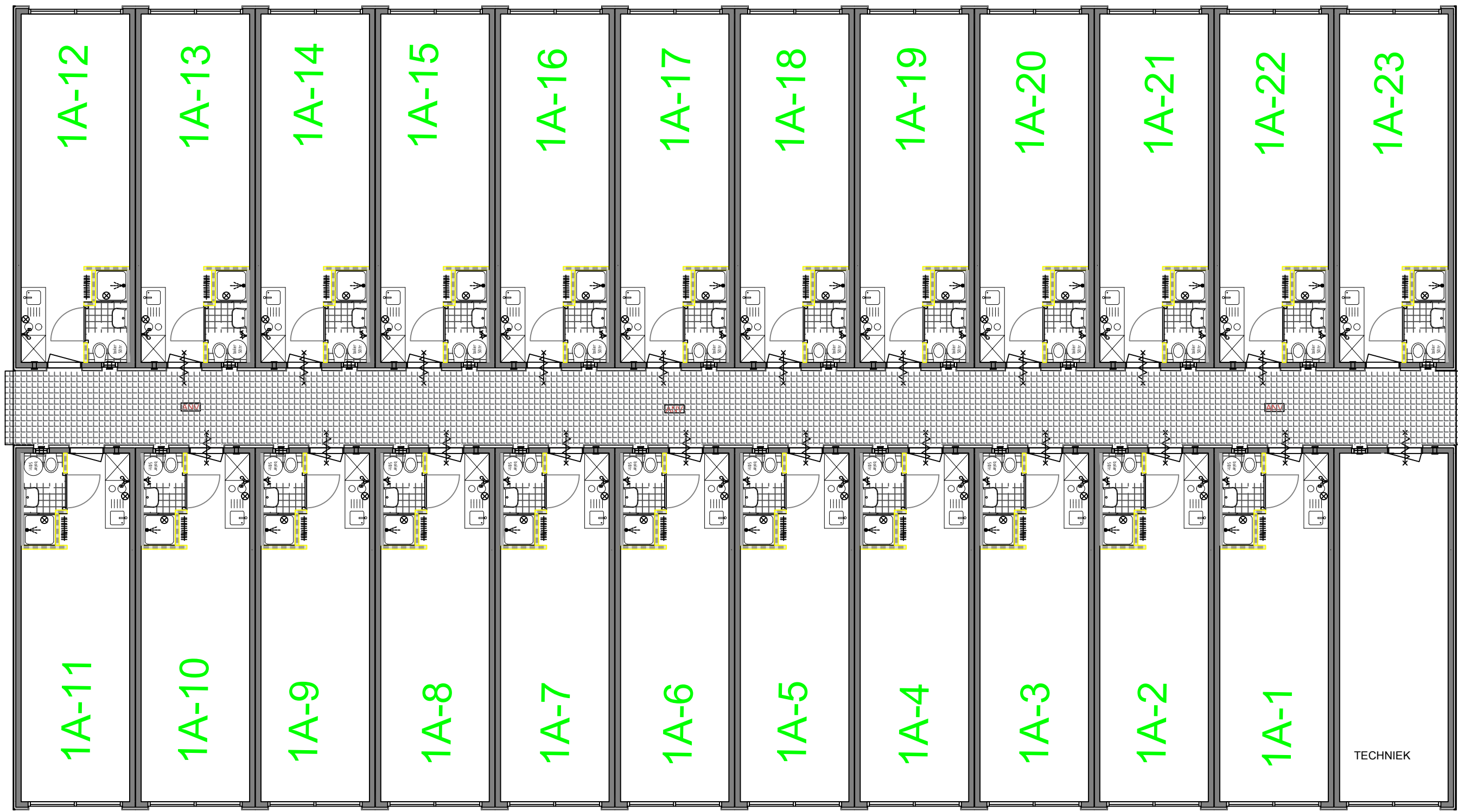
BEGANE GROND
